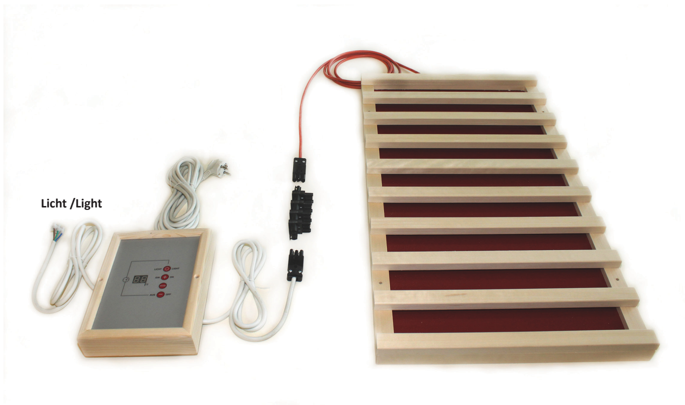
Variante B: Anschluss an Infrarot-Flächenheizung
